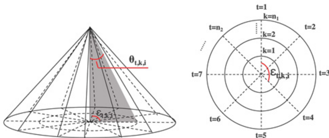
图 7: 锥形光线离散化示意图
