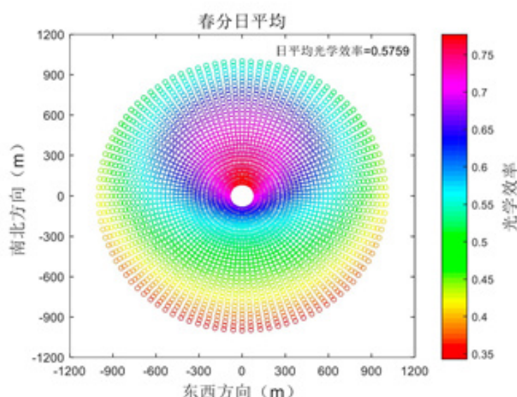
图 10: 春分日平均光学效率分布云图
