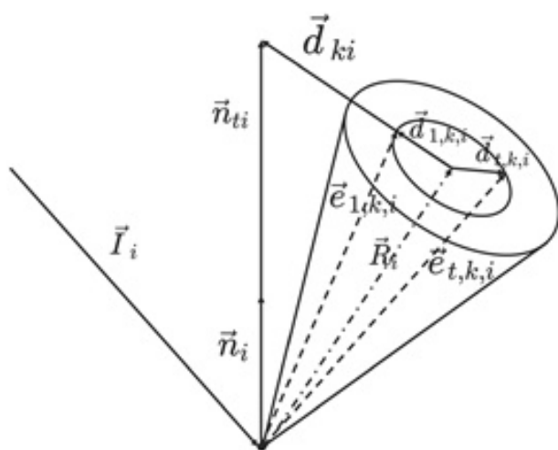
图 22: 离散光线向量 \vec{e}_{t,k} 计算示意图
